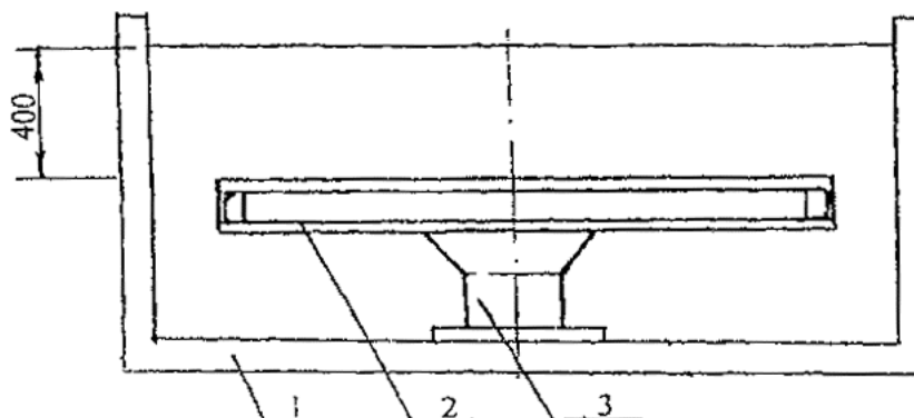
1 - емкость с водой; 2 - образец стеклопакета; 3 - вакуумная присоска
