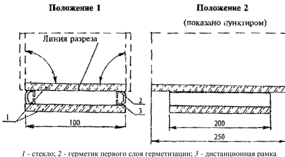
Рисунок 8 - Испытание герметика первого герметизирующего слоя
